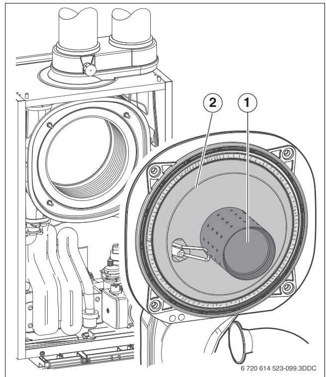
Afb. 38 Controleren isolatiedeel
