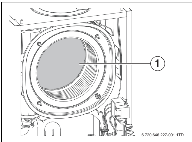
Afb. 35 Controleren isolatiedeel
