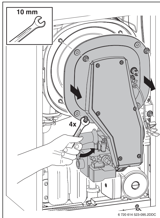
Afb. 33 Demonteren gas-luchtnit
