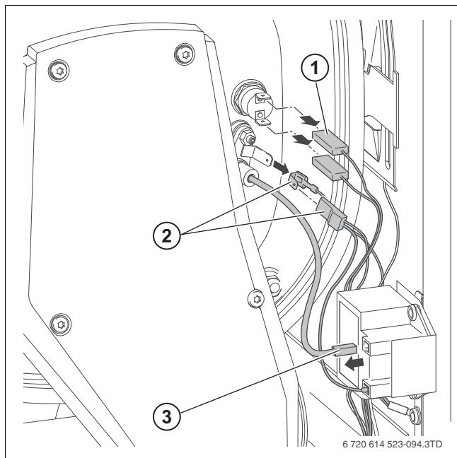
Afb. 31 Verwijderen stekkers gas-luchtnit
