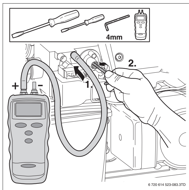
Afb. 43 Controleren gas-luchtverhouding
