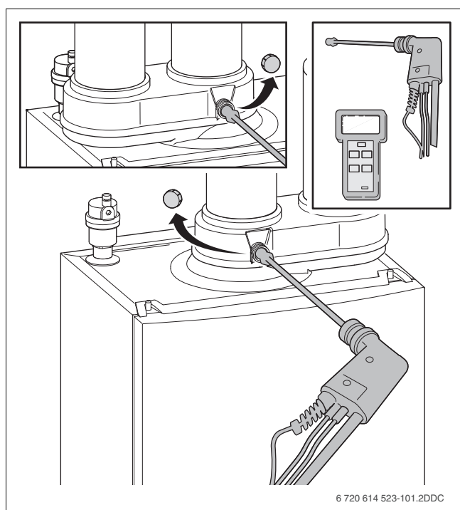
Afb. 46 Meten rookgaswaarden
