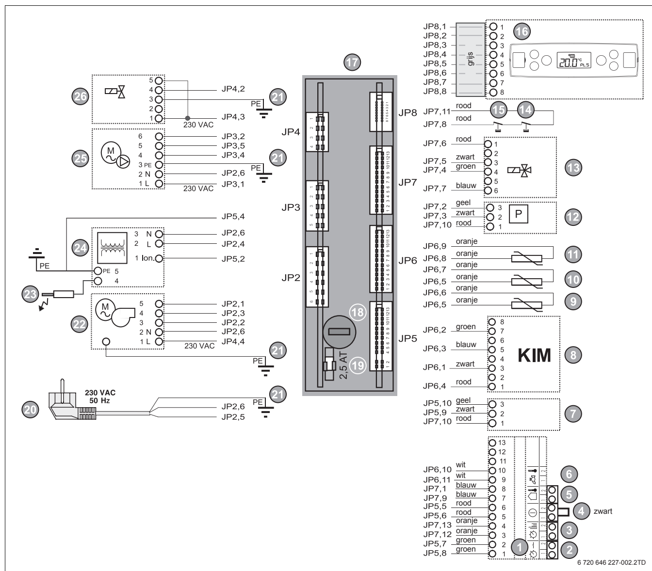
Afb. 5 Elektrisch schema
